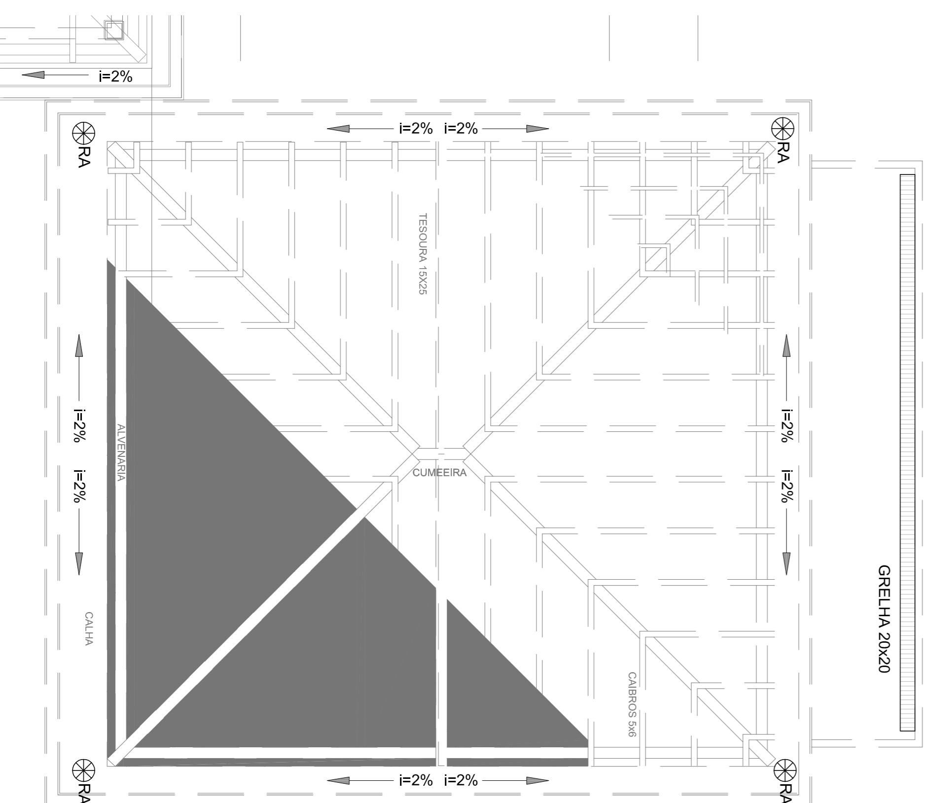
1 PLANTA BAIXA - PAV. TÉRREO ESCALA: 1/100
